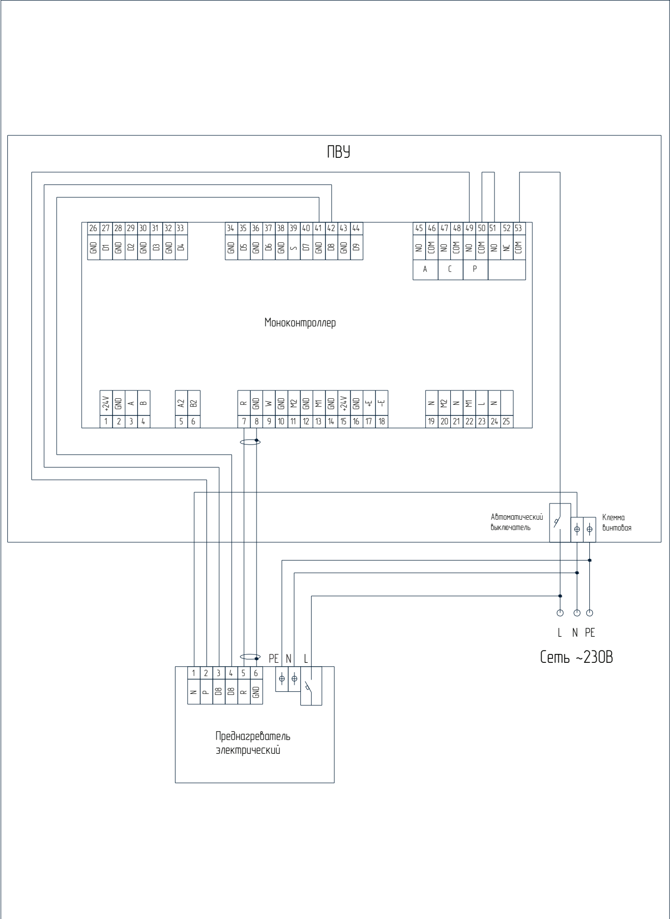
Подключение электрического преднагревателя (1 фаза) к моноконтроллеру ПВУ
