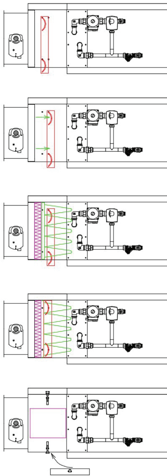
Установка двойной фильтрации
